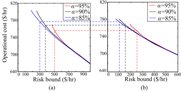
Fig. 6. (a) Efficient frontier at DS 1. (b) Efficient frontier at DS 2.
