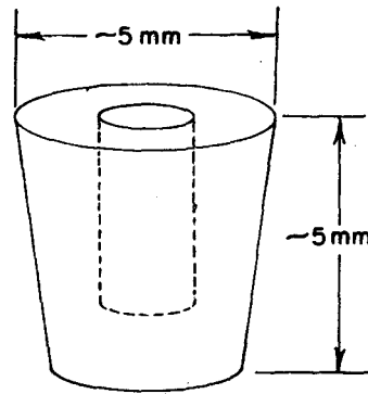
a. BaF_2 CRUCIBLE
