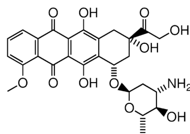
doxorubicin
