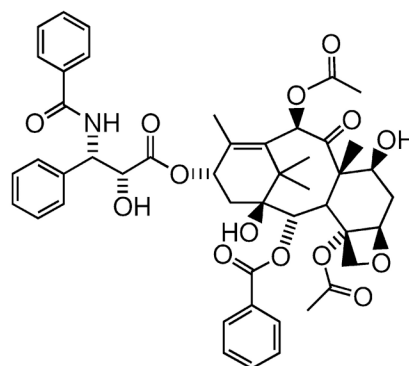
taxol
