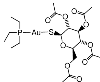
auranofin
