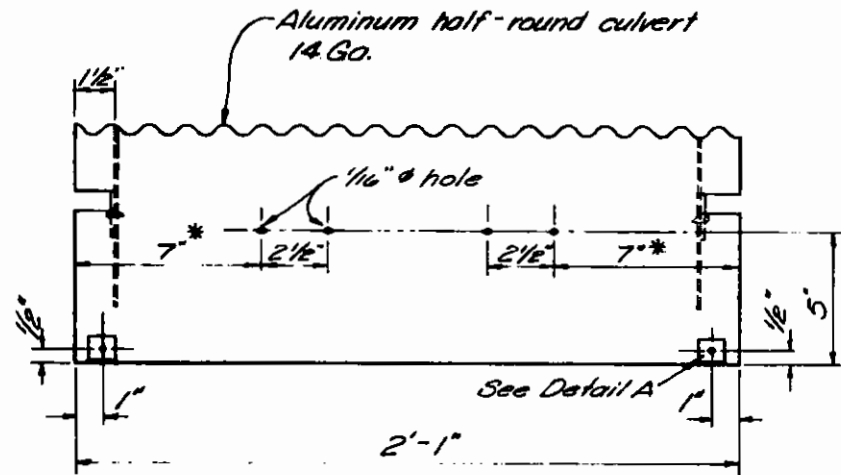
SIDE ELEVATION Scale: 3" = 1'-0"
