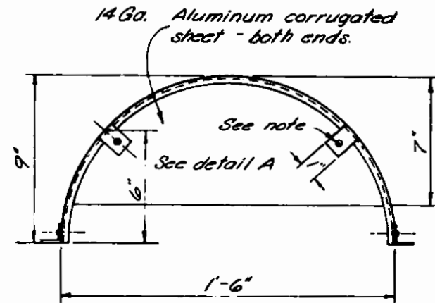
END ELEVATION Scale: 3" = 1'-0"
