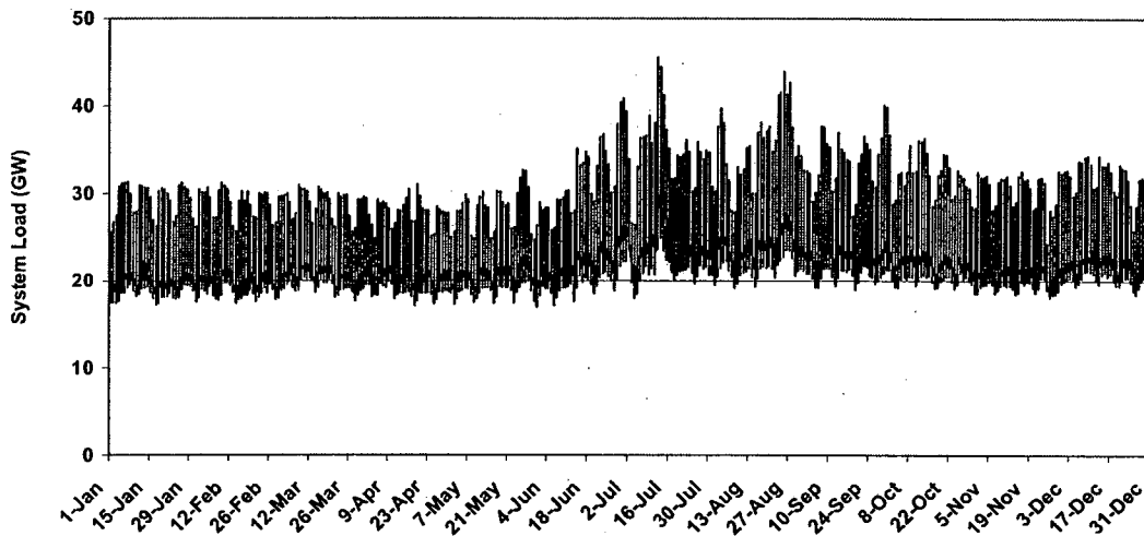
Figure 7. Actual 1999 CAISO Load
