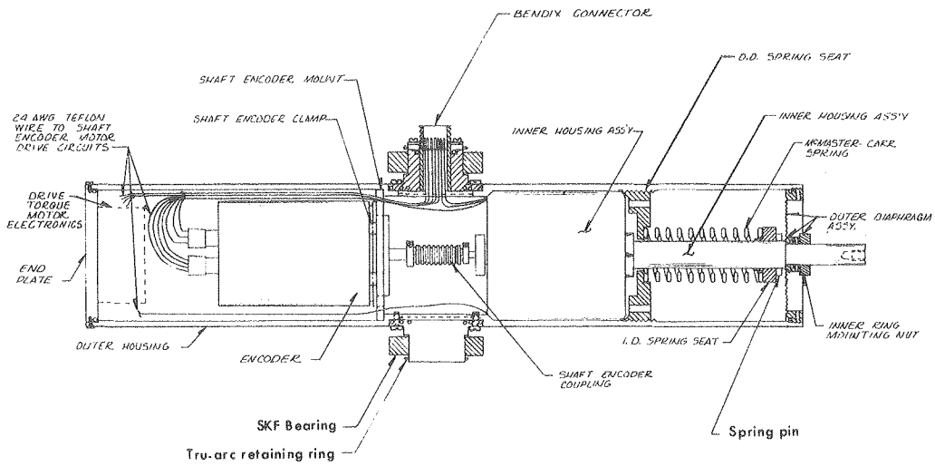
TMT PRECISION SERVO ACTUATOR SERVO ACTUATOR ASSY
