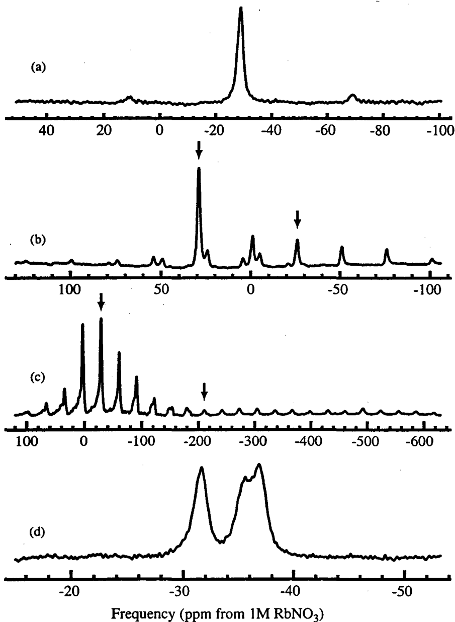
Figure 7.3 ^{87}\text{Rb} Salts 9.4T DAS Spectra. (a) \text{RbClO}_4 , (b) \text{Rb}_2\text{SO}_4 , (c) \text{Rb}_2\text{CrO}_4 , (d) \text{RbNO}_3 .
