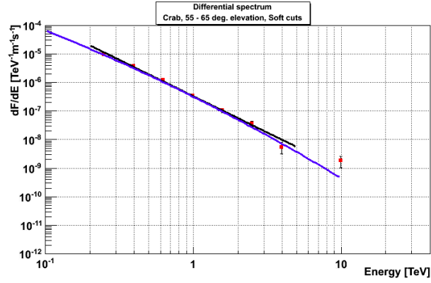
(b) 55^\circ > \text{Elevation} > 65^\circ
