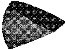
Edge blob \gamma - \alpha \leq \pi / 2
