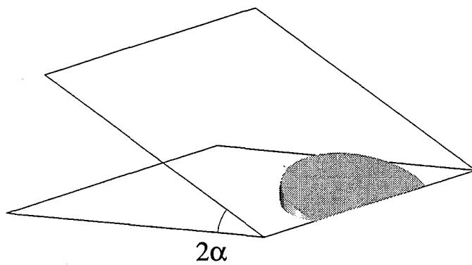
Figure 3. Edge blob
