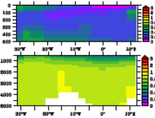
COBALT, GA-03
