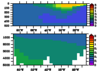
GENIE, GA-03
