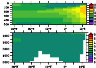
MITigsm, GA-03
