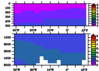
GENIE, GA-03
