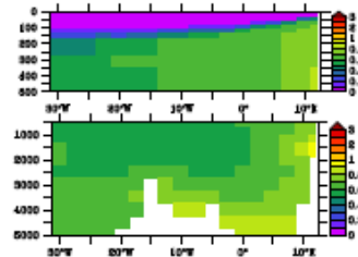
PISCES 2, GA-03
