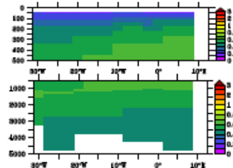
MITecco, GA-03
