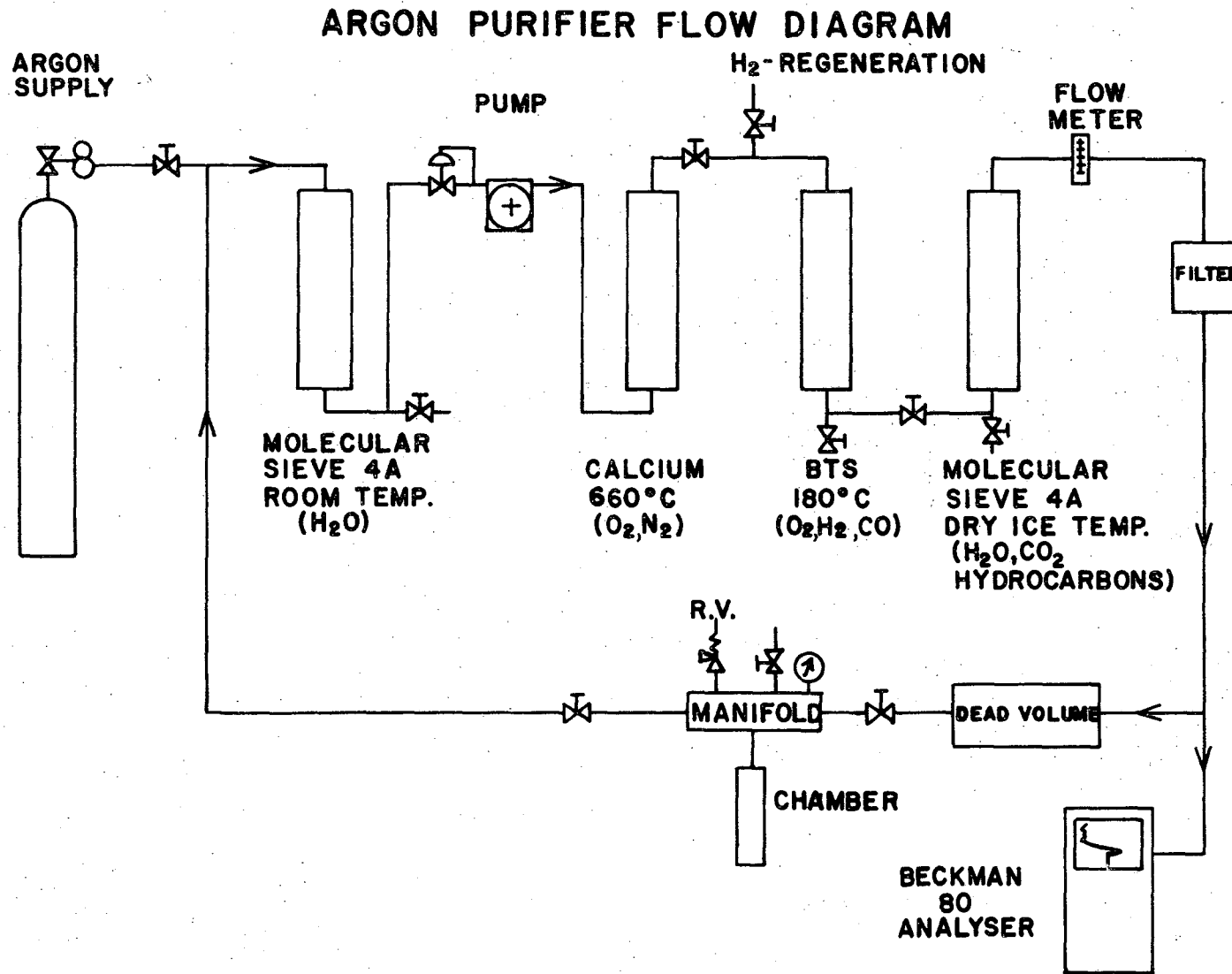
Fig. 3. Argon purifier.
