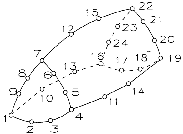
16. CUBIC SOLID WEDGE
