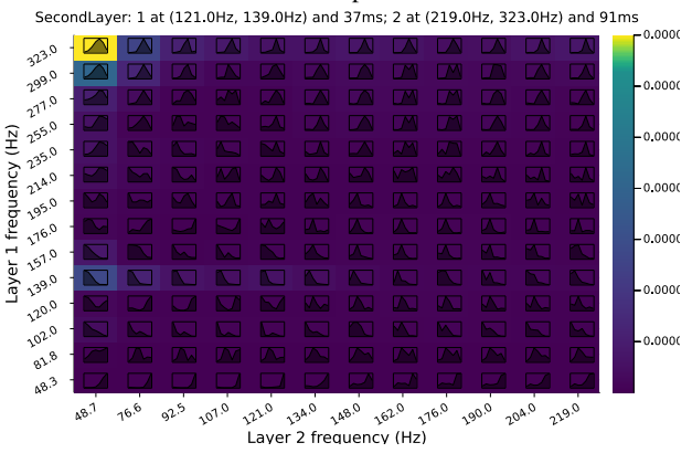
(d) The second layer coefficients of Fig. A.8b
