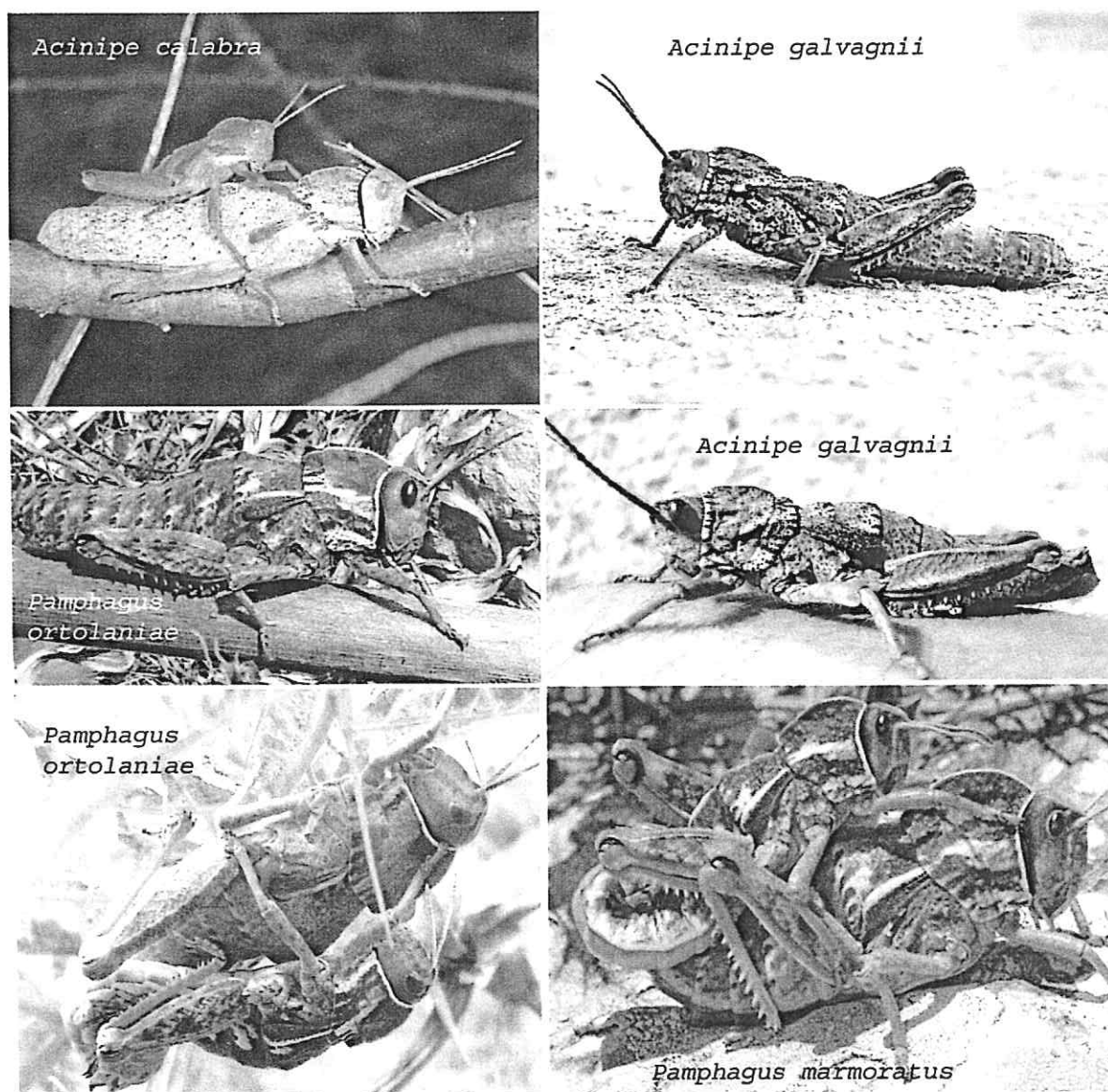
Tavola 4 – Pamfagidi di Sicilia. Acinipe calabra è specie calabro-siculo-maghrebina, Acinipe galvagnii , Pamphagus marmoratus e Pamphagus ortolaniae (Lampedusa) sono endemici. Dall'alto a sinistra in basso a destra, foto di A. Falci, T. Puma, B. Massa, F. Marrone, B. Massa, R. Kleukers.
