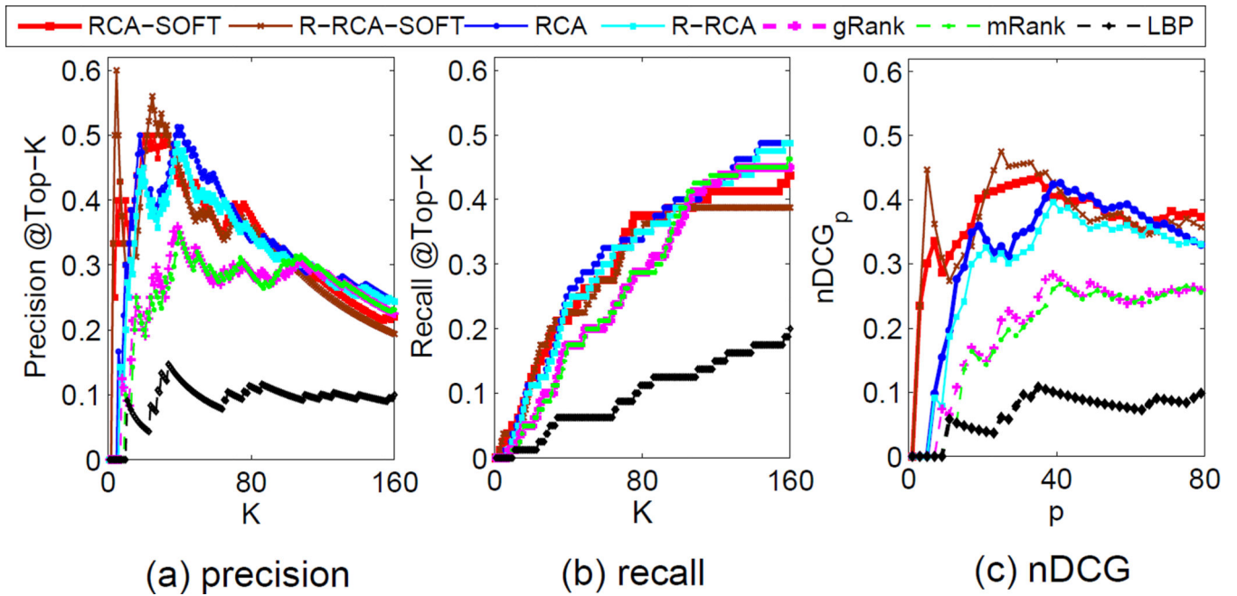
Figure 6. Comparison on BIS data.
