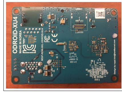
(b) Odroid XU-4 back
