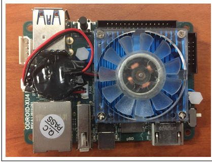
(a) Odroid XU-4 front
