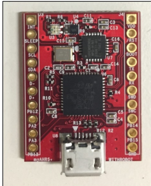
(a) myAHRS+ IMU sensor
