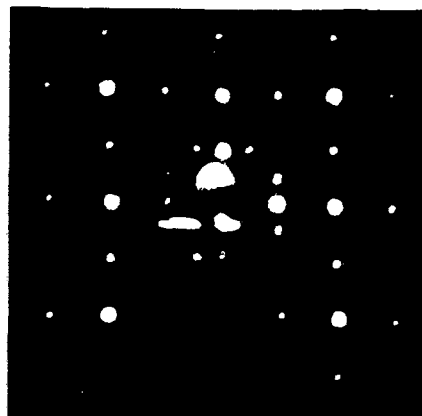
c(4x2) - LEED Pattern
