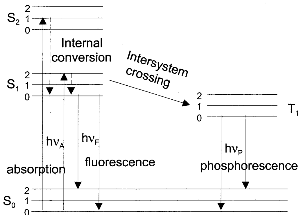
Fig.1.1. Jablonski diagram.
