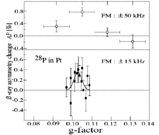
Fig. 2. NMR spectra.
