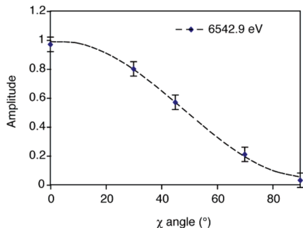
(a) Mn-nitrido
