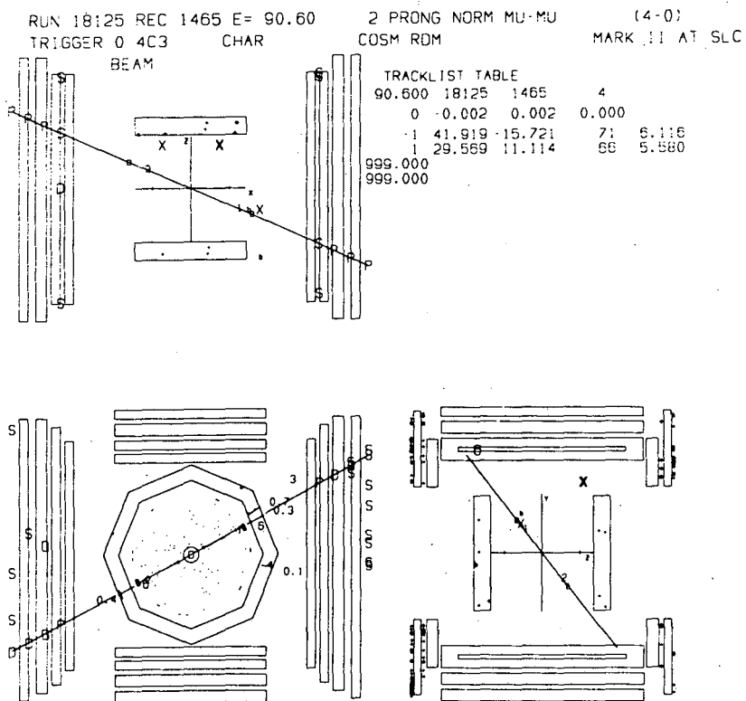
Fig. 21. A \mu^+\mu^- candidate.
