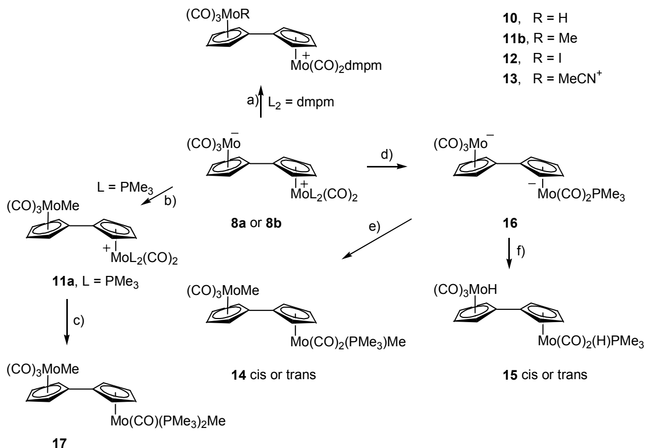
Scheme 4 a) 8b + HBF 4 ·Et 2 O → 10 ; 8b + CF 3 SO 3 Me → 11b ; 8b + I 2 → 12 ; 8b + AgBF 4 → 13 . b) MeI. c) LiAlH 4 . d) Na/Hg. e) MeI. f) CF 3 COOH.
