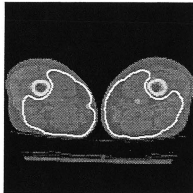
(d) t = 0.6000
