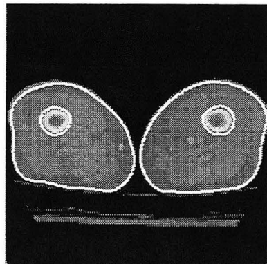
(f) t = 1.6000
