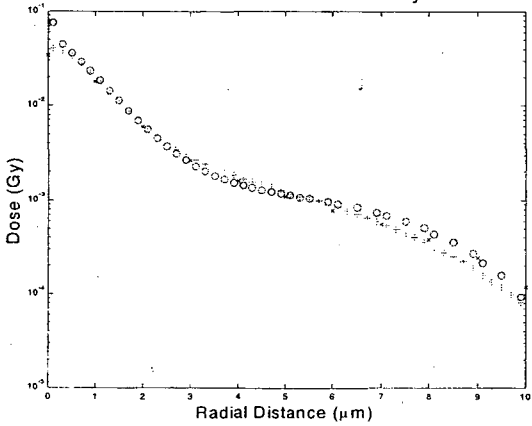
PENELOPE - MCNP - PITS: Layer 4
