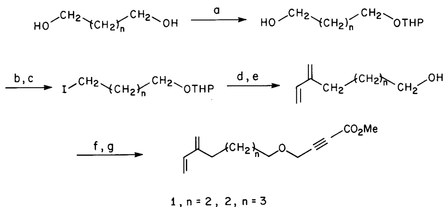
Scheme 1. (a) DHP, H + ; (b) MsCl, Et 3 N; (c) NaI, acetone, reflux; (d) CH 2 CHC(MgCl)CH 2 , THF, Li 2 CuCl 4 ; (e) H 3 O + ; (f) NaH, DME, HCCCH 2 Br; (g) n-BuLi, ClCO 2 CH 3 .
