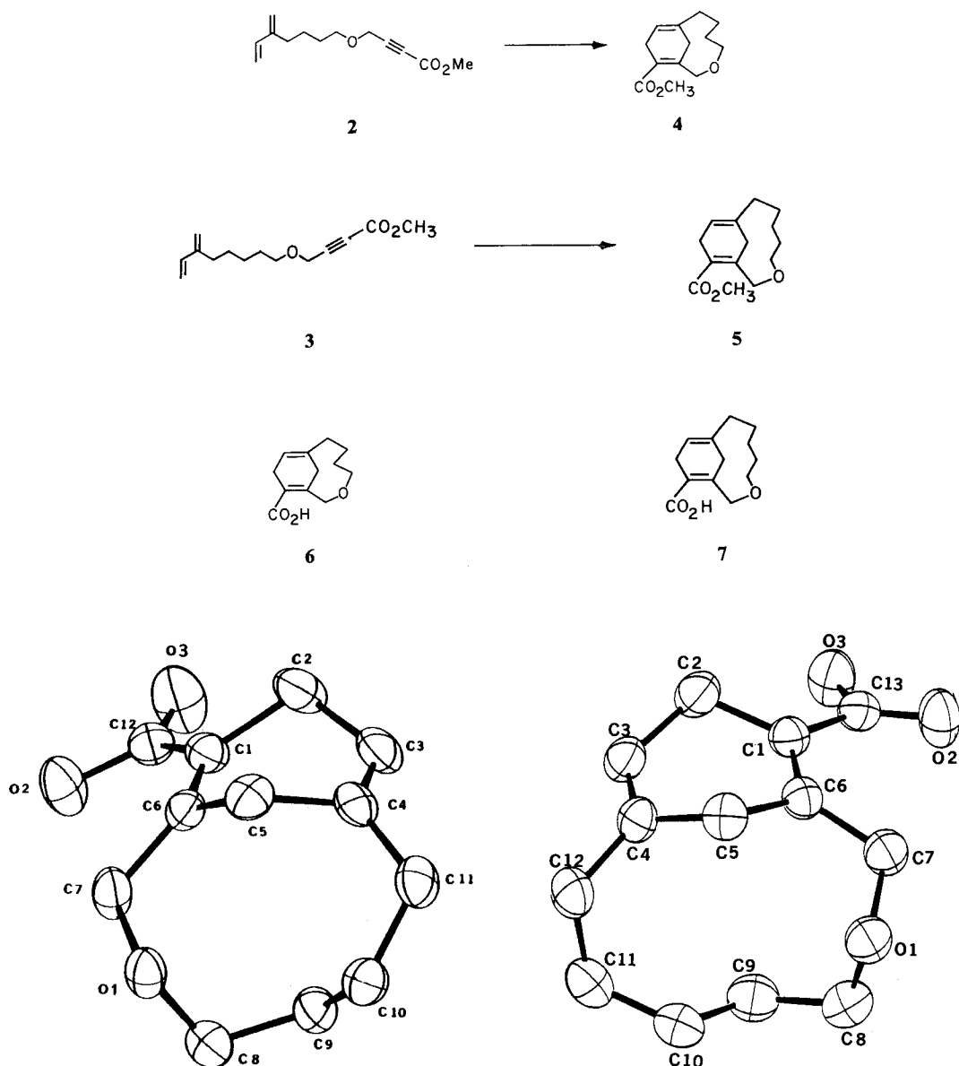
Scheme 1. (a) DHP, H + ; (b) MsCl, Et 3 N; (c) NaI, acetone, reflux; (d) CH 2 CHC(MgCl)CH 2 , THF, Li 2 CuCl 4 ; (e) H 3 O + ; (f) NaH, DME, HCCCH 2 Br; (g) n-BuLi, ClCO 2 CH 3 .
