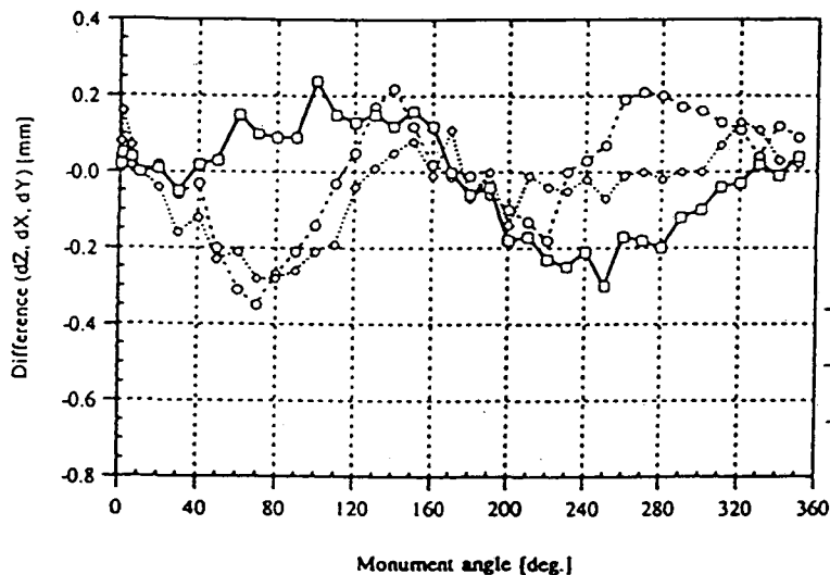
Figure 7 ALS Storage Ring monument Changes from 1/95 to 8/95
