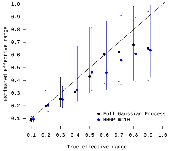
(d) \sigma^2 = 0.5
