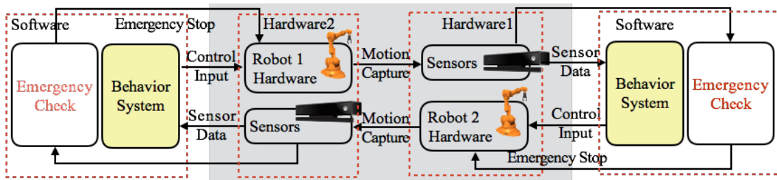
(d) Robot-robot interaction platform.
