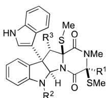
R 3 = OH [ gliocladin A/bionectin C: R 1 , R 2 = H (11) T988 B: R 1 = CH 2 OH, R 2 = H (12) oidoperazine A: R 1 = CH 2 OH, R 2 = CHO (13) R 3 = H [ gliocladin B: R 1 , R 2 = H (14)
