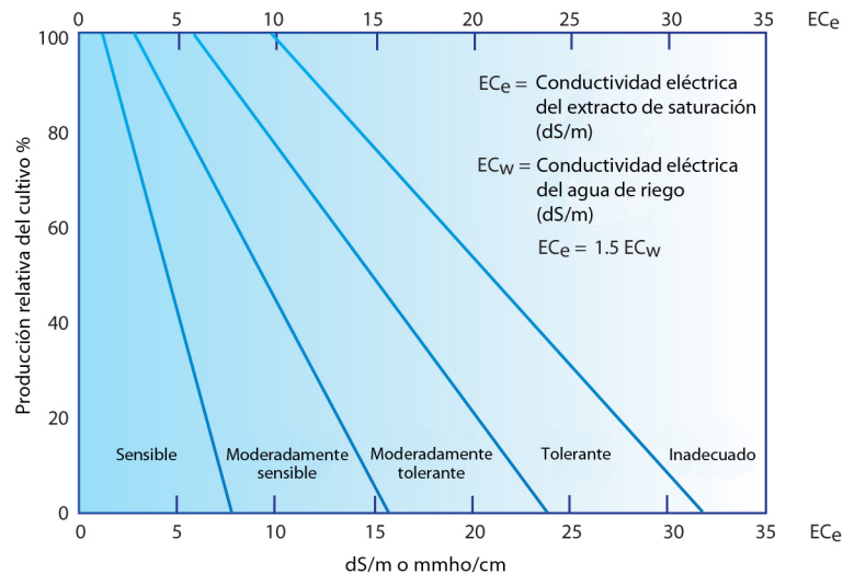
Figura 2. Producción relativa de un cultivo (o potencial productivo) en función de la salinidad promedio de una zona de raíces ( EC_e , dS/m) agrupada de acuerdo con la tolerancia relativa o sensibilidad a la salinidad. Fuente: adaptado de Maas and Grattan 1999; Grieve et al. 2012).
