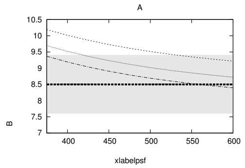
(d) Total (NP+SM) t\bar{t} production
