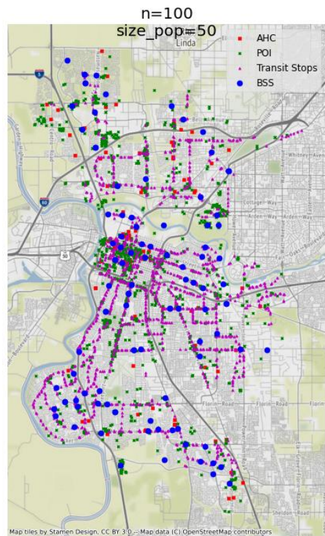
d) n=100
