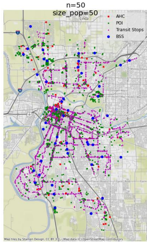
b) n=50
