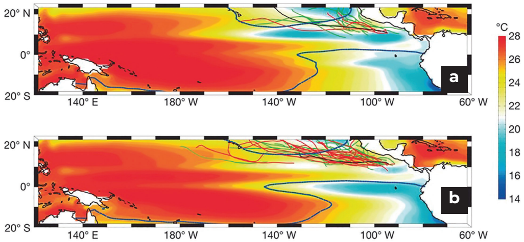
Figura 6: Temperatura subsuperficial de verano (junio-noviembre) promediada durante los períodos en A) PC2 < -1 desviación estándar y, B) cuando PC2 > 1 desviación estándar. La línea azul gruesa denota la isoterma de 26 °C de la temperatura superficial del mar promediada durante los períodos de baja (A) y alta (B) actividad de PC2. En cada panel, las líneas coloreadas representan las trayectorias de los ciclones tropicales fuertes que ocurrieron durante los períodos correspondientes: verde = categoría 3; rojo = categoría 4; negro = categoría 5 en la escala Saffir-Simpson. Figura tomada de Jin et al. (2014).
