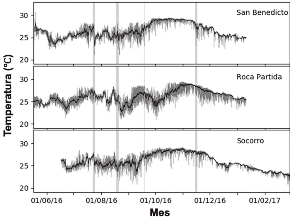
Figura 10: Remperatura registrada diariamente in situ con termómetros HOBO en las islas San Benedicto (23 m de profundidad), Socorro (28 m) y Roca Partida (38 m). Datos observados (gris) a intervalos de 13 minutos y promedio diario móvil (línea negra). Las barras verticales sombreadas indican períodos cuando ciclones tropicales estuvieron dentro de un radio de 200 km de las islas (Carter et al., 2020).
