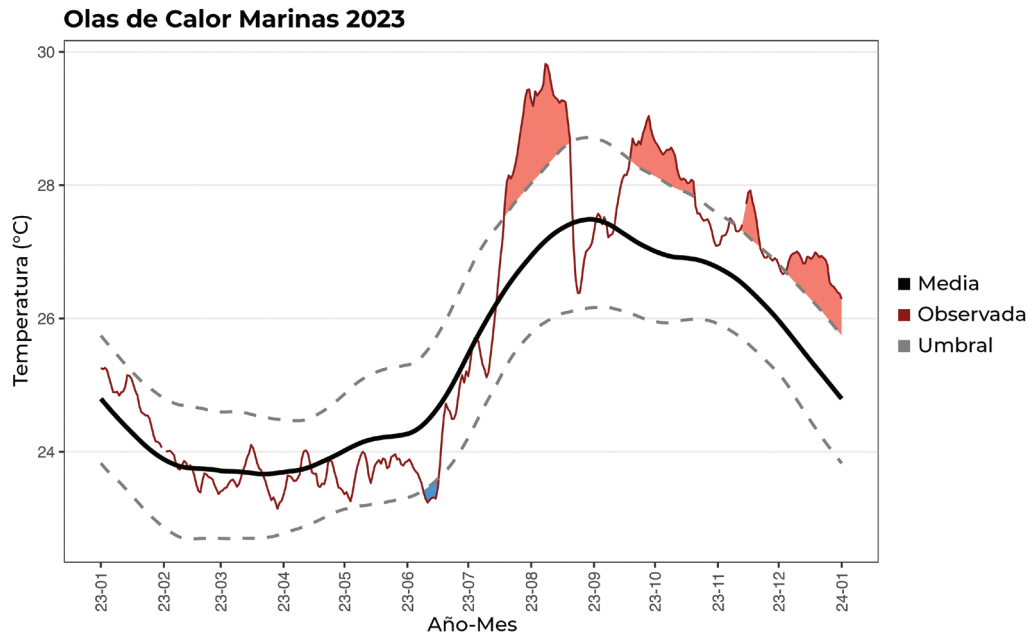
Figura 17: Olas de Calor Marinas inferidas al exceder el umbral de una desviación estándar ocurridas en el Archipiélago de Revillagigedo durante el año 2023. La línea sólida negra define el promedio climatológico, proporcionando una base contra la cual se miden los umbrales. Las líneas discontinuas indican el umbral para las condiciones de ola de calor, típicamente definidas como temperaturas que están a una desviación estándar por encima del promedio histórico. La línea roja traza la temperatura observada para 2023, con áreas sombreadas en rojo resaltando las instancias donde las temperaturas observadas superan el umbral, definidas como olas de calor marina.
