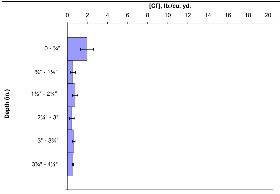
Figure 65. Chloride profile for SR 82 MP 43.524 (Wapato).
