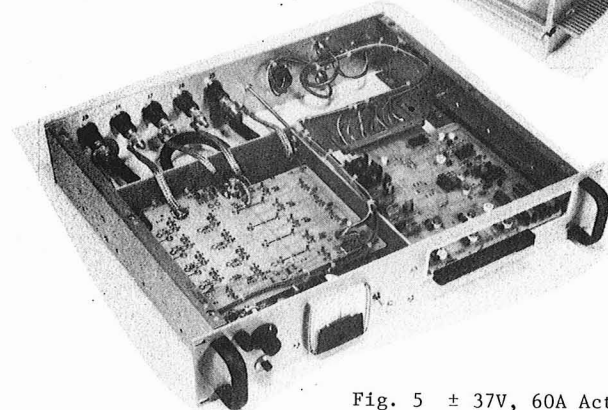
Fig. 5 \pm 37 V, 60A Actuator
