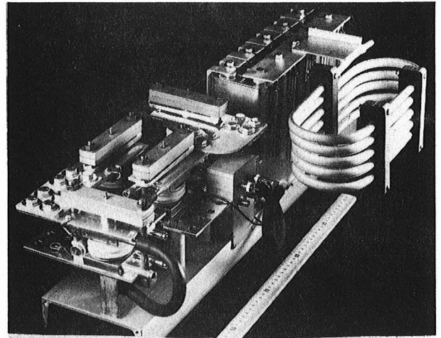
Fig. 2 400 amp Chopper Module
